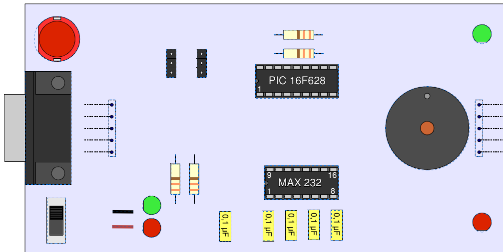
Orni RS V2 : Implantation des composants
